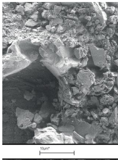
Observe la calidad de su producto – análisis SEM (microscopio electrónico de barrido) de lodos de perforación
