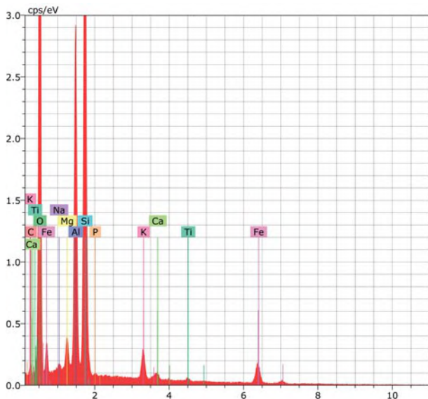
Análisis de pruebas utilizando la técnica EDX (espectroscopia de rayos x por dispersión de energía)
