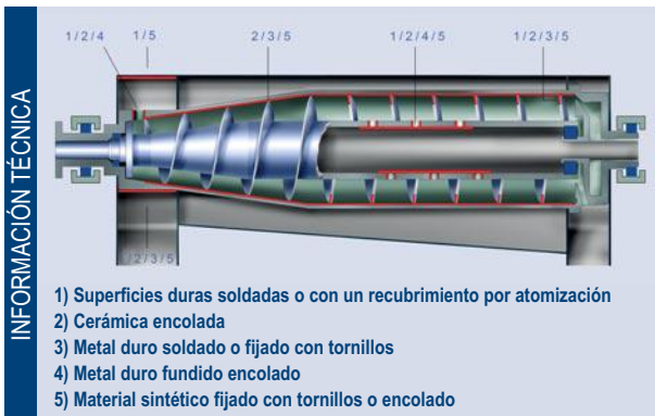
Elementos reemplazables de la protección antidesgaste
