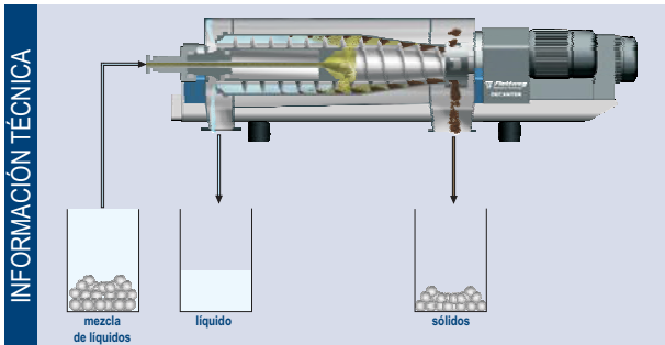
Flujo de los líquidos y de los sólidos en un Decanter Flottweg
