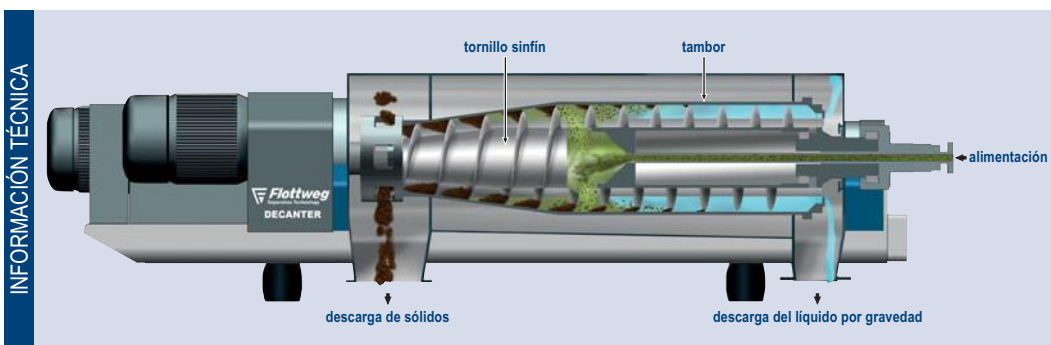
Decanter Flottweg para la separación de sólidos suspendidos en un líquido con descarga de la fase líquida (centrado) por gravedad
